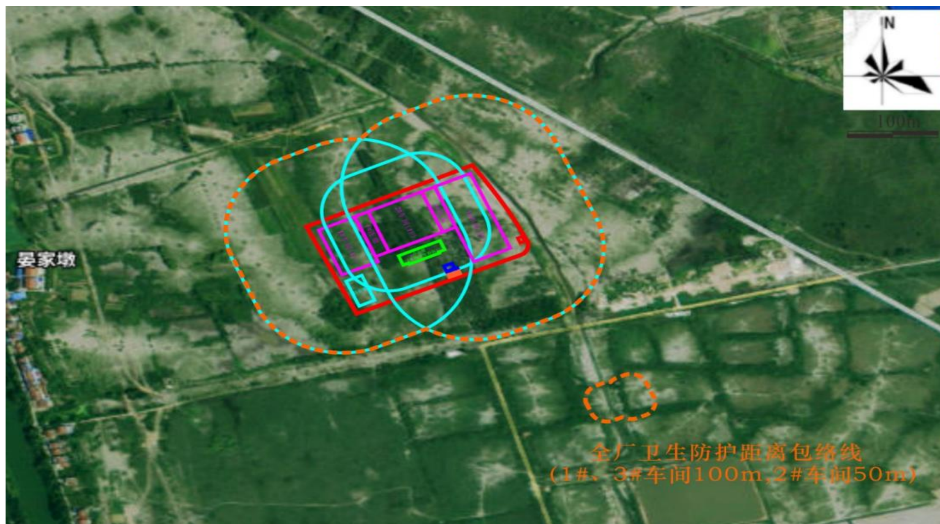
附图 11 项目卫生防护距离包络线图
