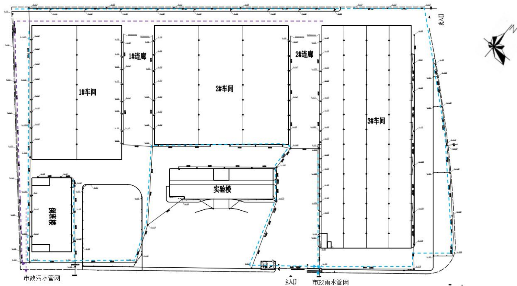
附图 8 项目厂区雨污管网图
