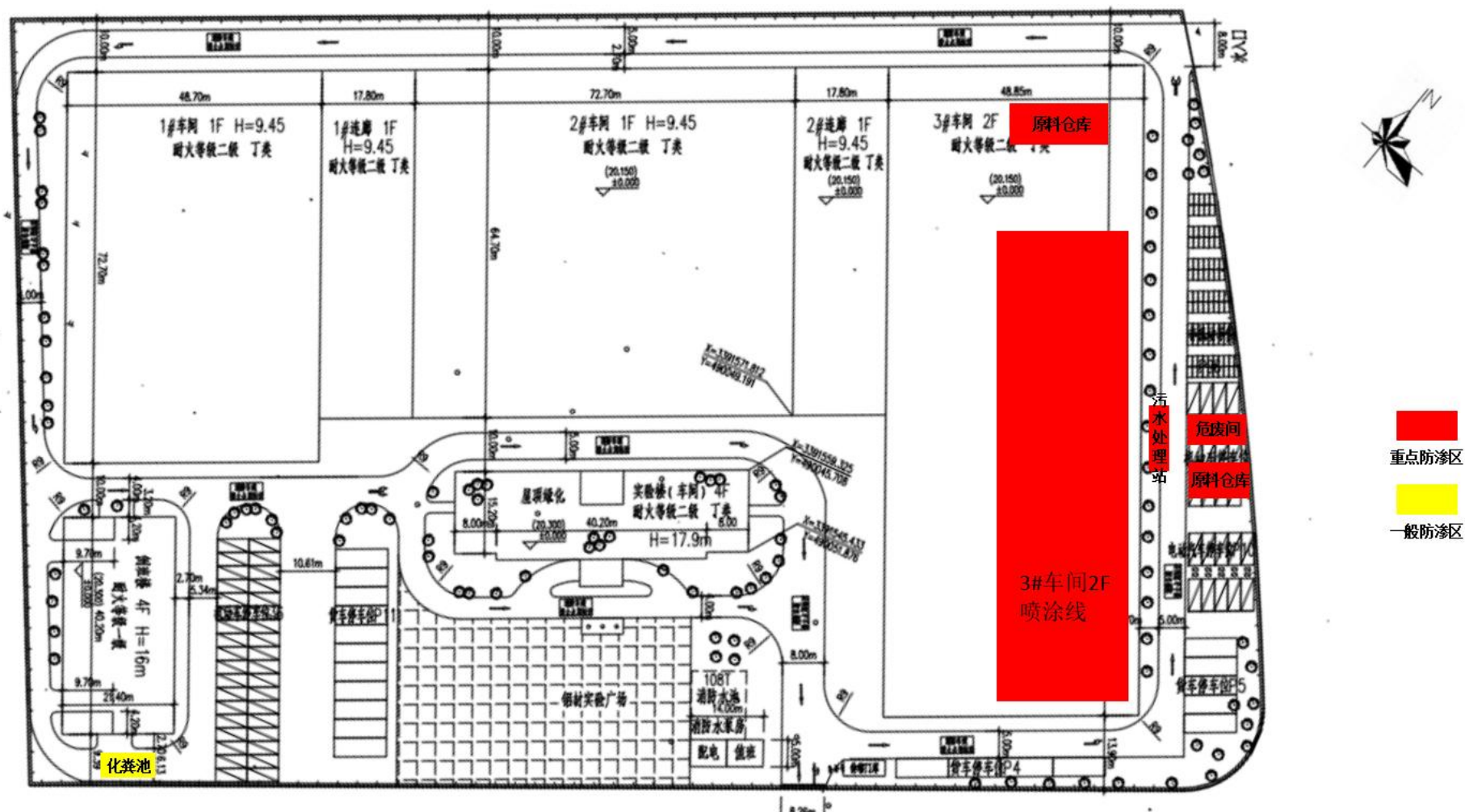
附图9 项目分区防渗图
