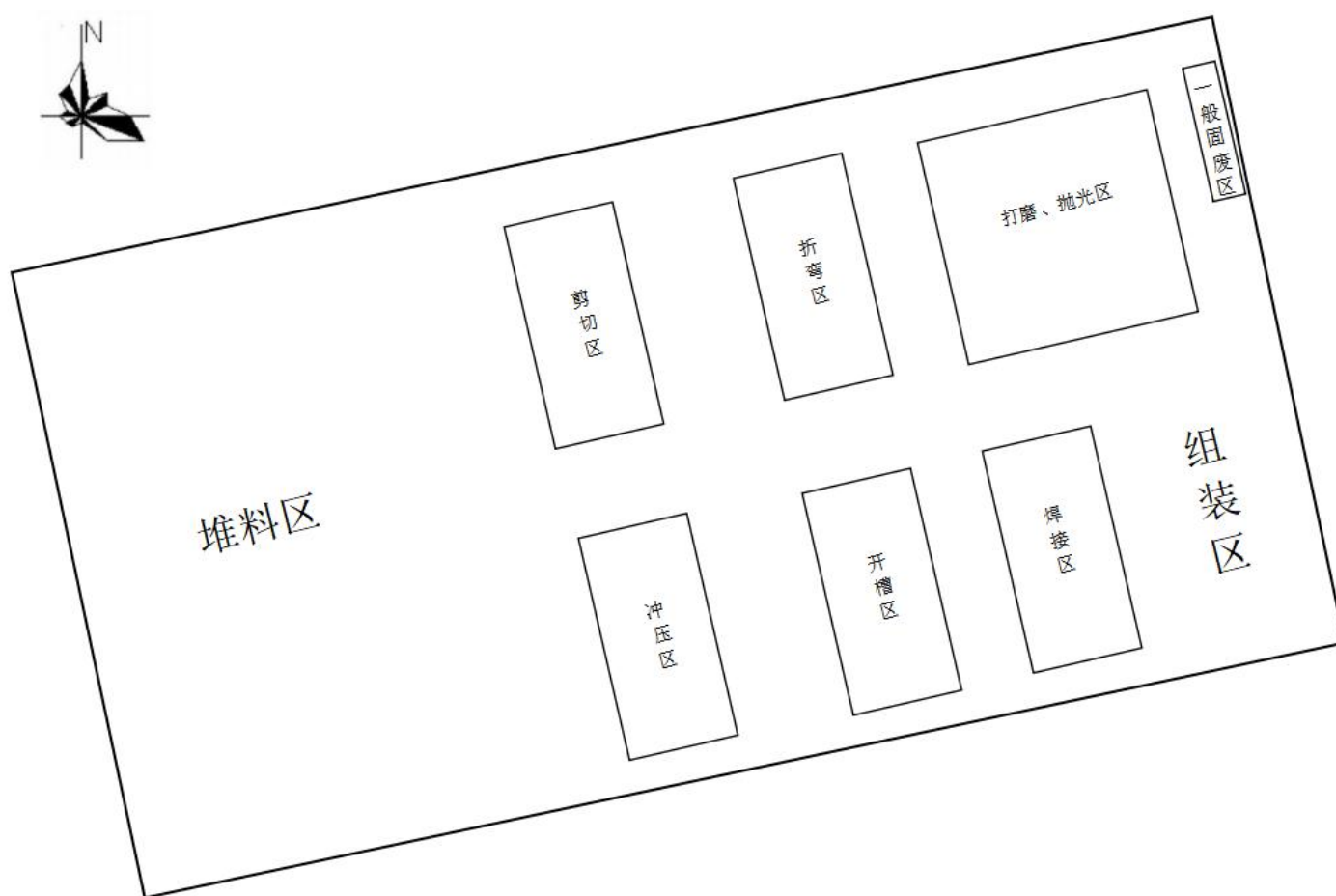
附图 5 项目 2#车间平面布置图
